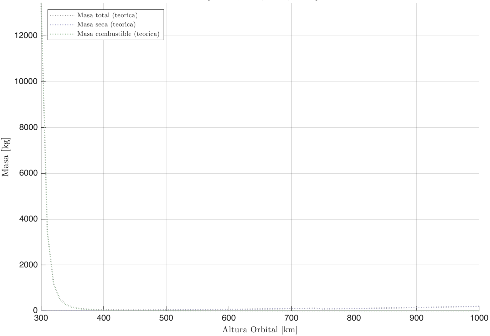
Desglose de Masas vs. Altura Config: 1 Sat, 2 Tel, Det 1, Cassegrain
